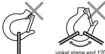
Forkert placering af krogen på den løftede last eller slyngen
