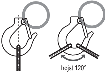
Slyng lasten med krogakslens forlængede linje.
