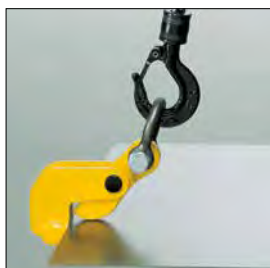
THK Klo Bæreevne: 0,75 – 9,0 ton Anvendes parvis for løft af plader
